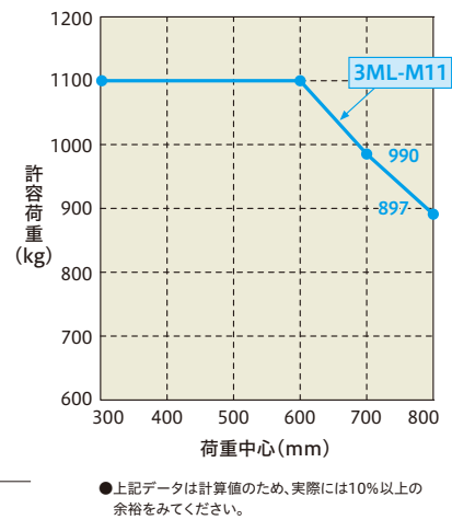
サイドフォーク荷重データ
